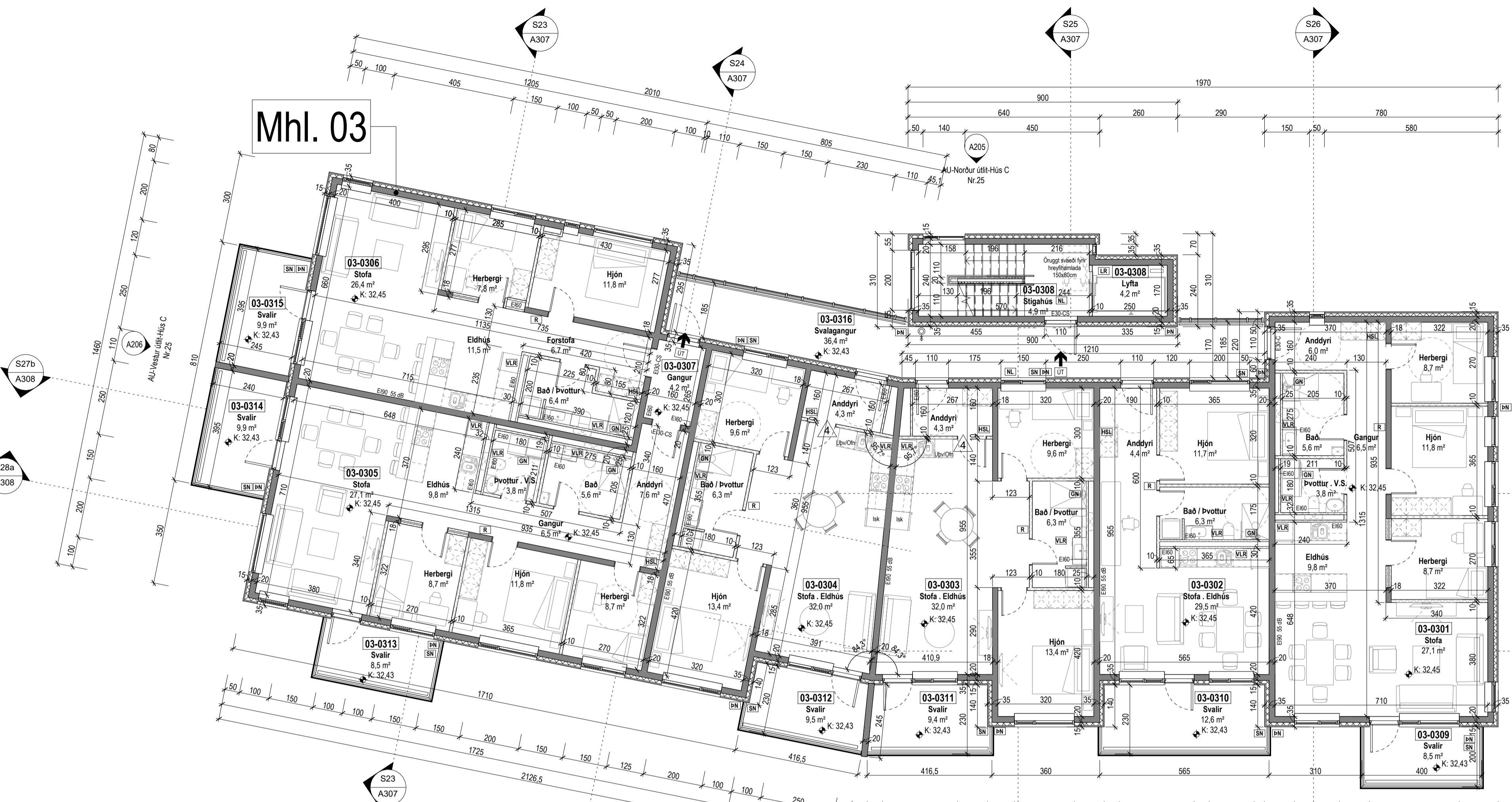
Grunnmynd 3.hæð 1:100
