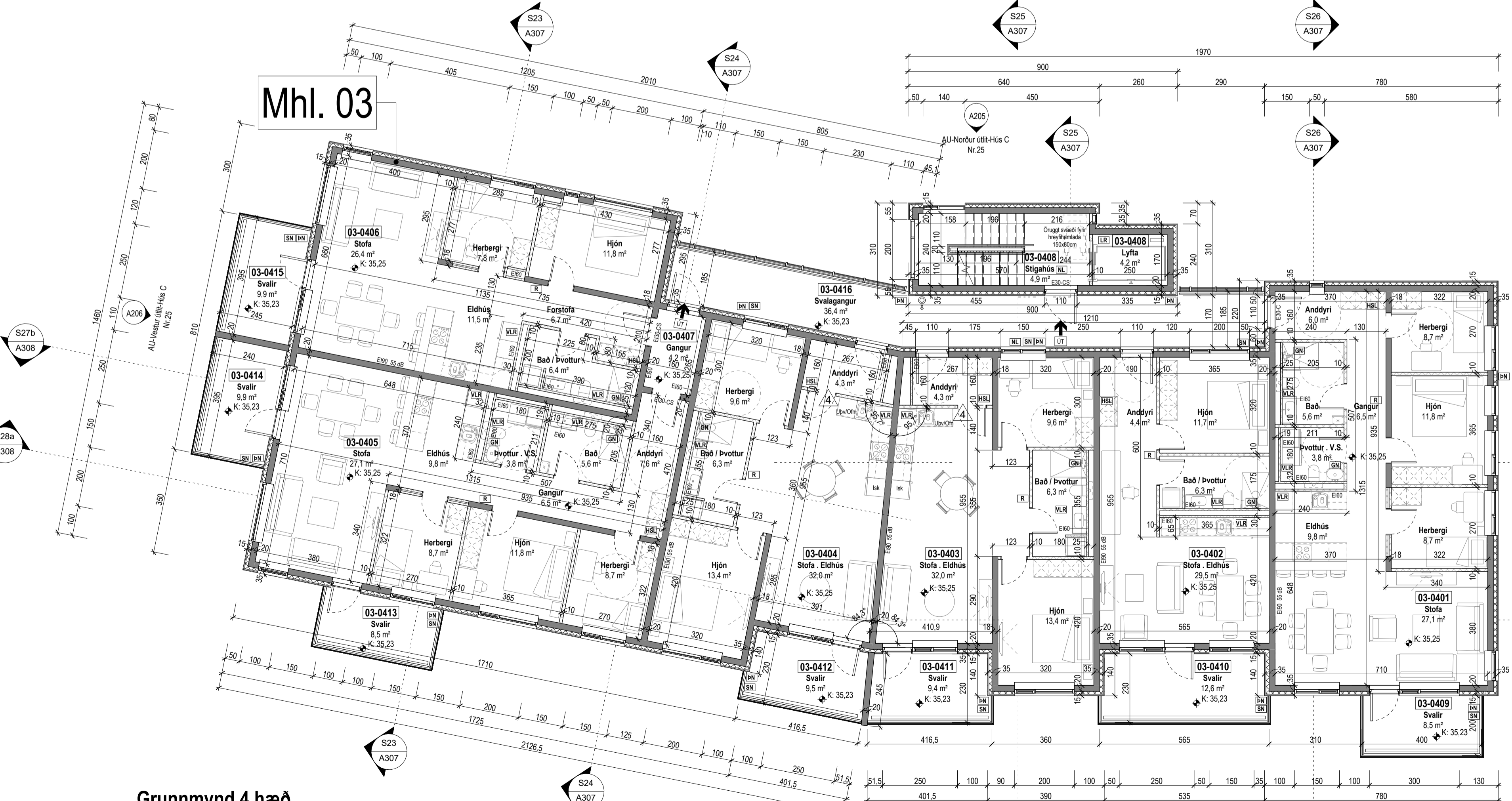
Grunnmynd 4.hæð 1:100
