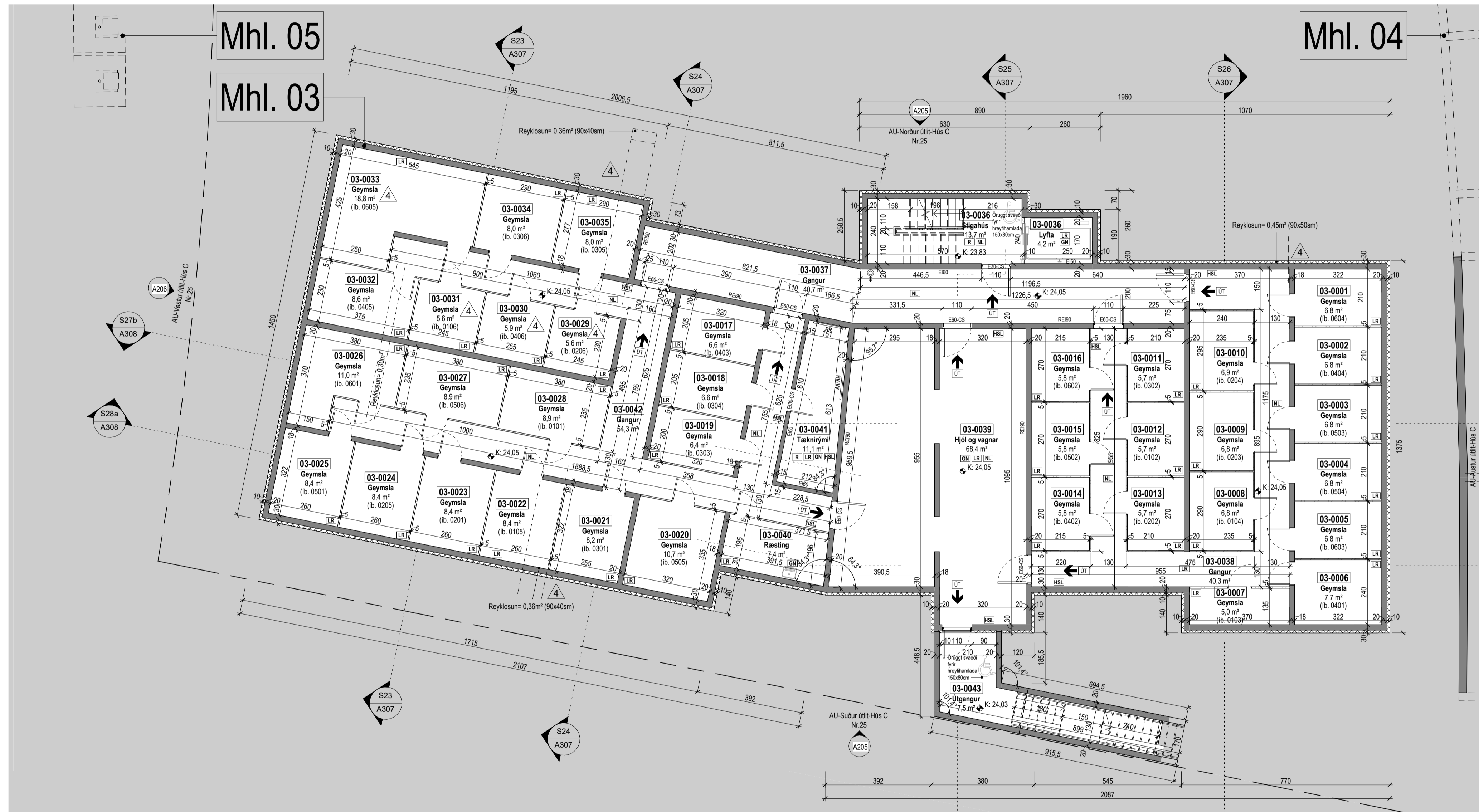
Grunnmynd kjallara 1: 100
